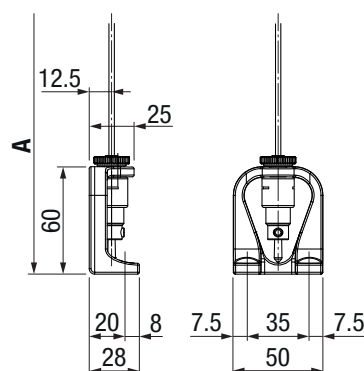
Support au sol VA201-1
