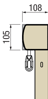
Montage en embrasure
