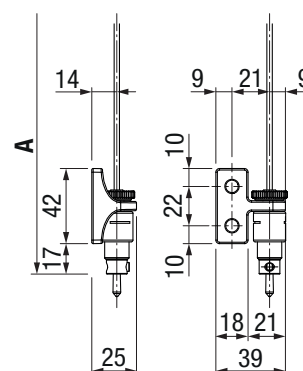
Support en embrasure VA214-1
