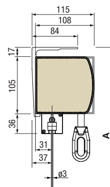
Console sous dalle plate VA210-1
