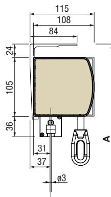
Console sous dalle haute VA211-1
