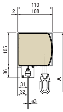
Console murale VA221-1
